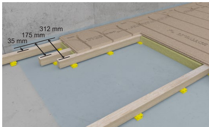
Figur 4 Klimagolv med kantregel cc. 35 mm från vägg och med extra regel under vändspår och under skarv mellan vändplattor och golvskivor, se monteringsanvisningen för Kronospan vändplattor. Där vändplattor inte används, skall vändspåren fräsas i Klimagolvets. Vändspår skall understödjas 200 mm från vägg, se figur 2.
